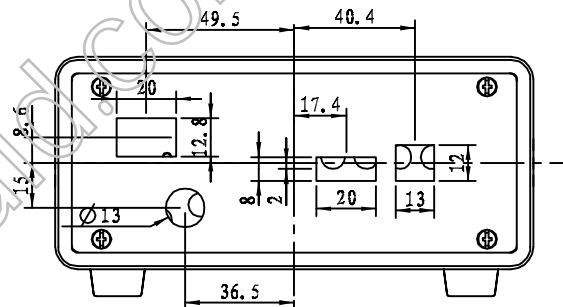
后视图
