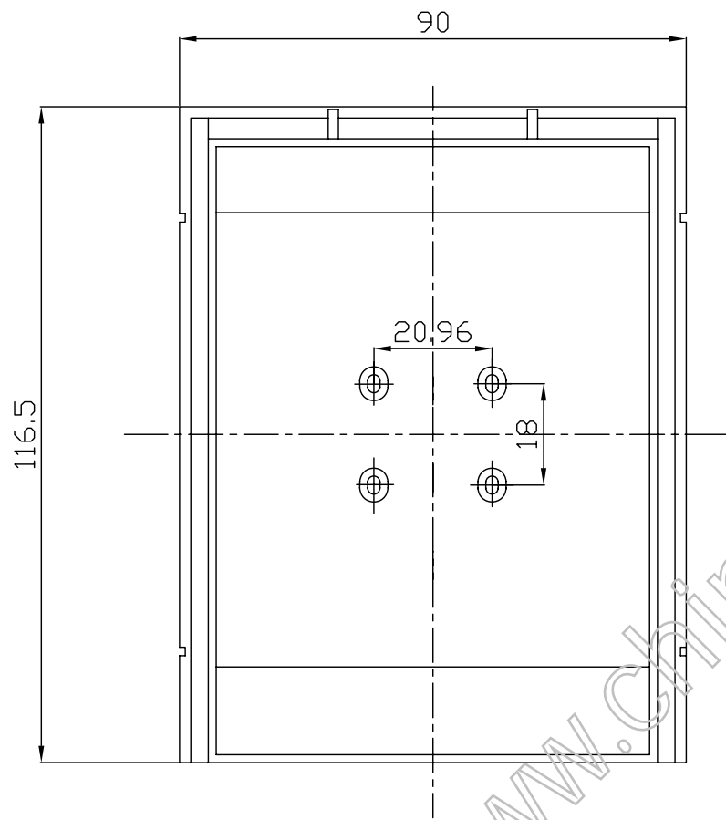
上盖反面视图
