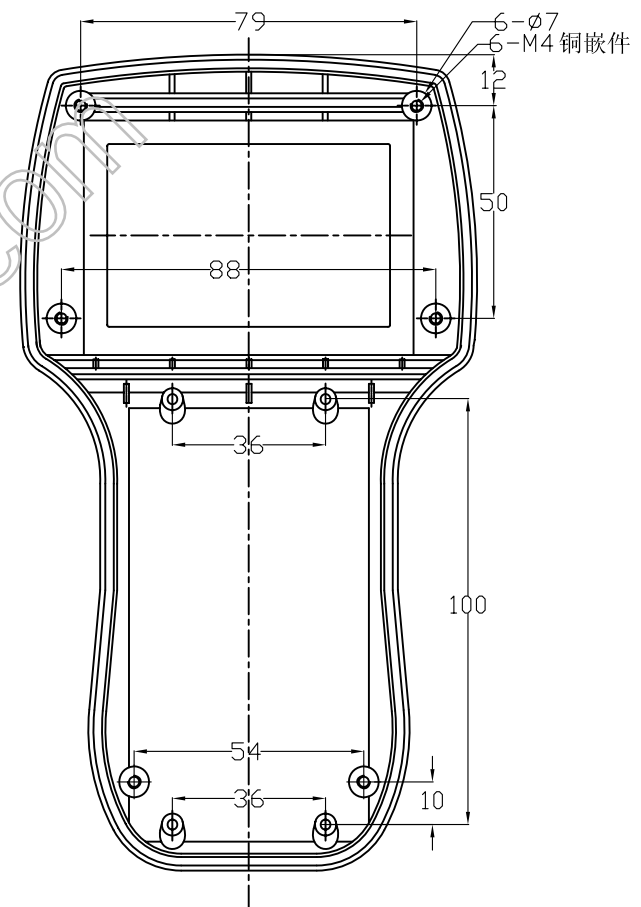
上盖底视图
