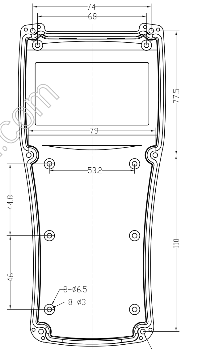
上盖底视图
