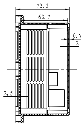
截面 A-A
