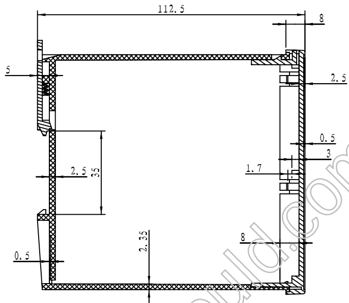
前面 A-A
