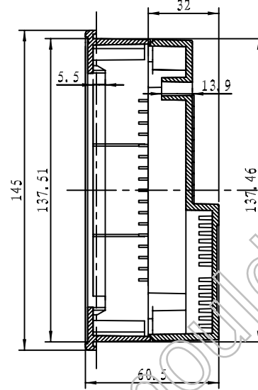
剖面 A-A
