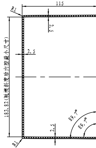
剖面 A-A
