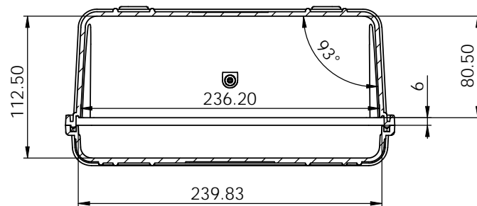
剖面 B-B
