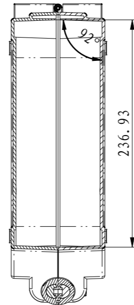
截面 A-A
