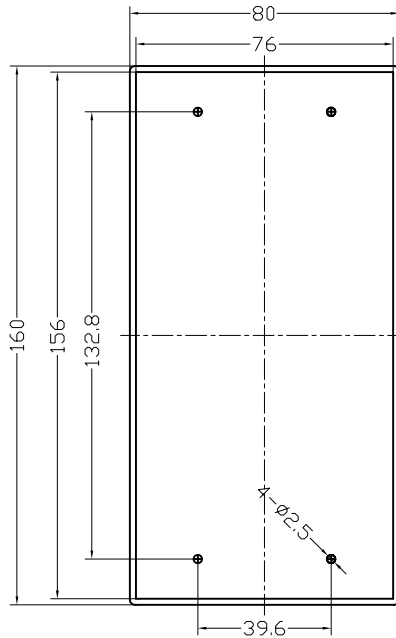
面框正视图
