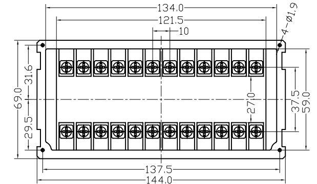
(2) 插式接线板图
